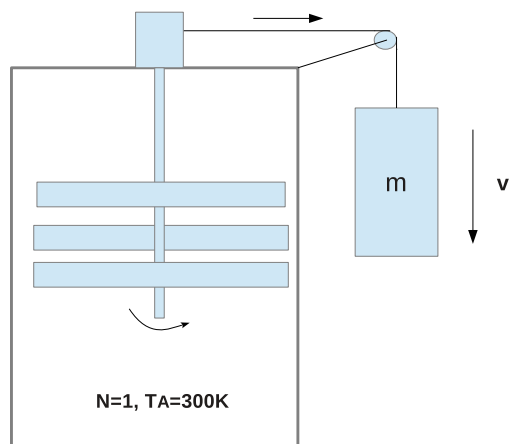
Figura 1: (Ejercicio 1) la masa m desciende y el movimiento se transmite por la soga y un mecanismo de engranajes a un paleta que agita al gas.
