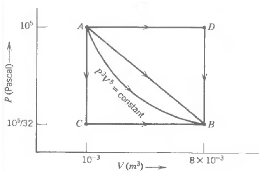
Figura 2: Estados y procesos para los Problemas 5 y 6 ; la curva convexa que une los puntos A con B es la adiabática P^3V^5 = cte .
