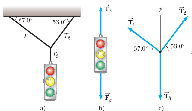
Figura 5.10 (Ejemplo 5.4) a) Un semáforo suspendido por cables. b) Diagrama de cuerpo libre del semáforo. c) Diagrama de cuerpo libre del nudo donde se juntan los tres cables.
