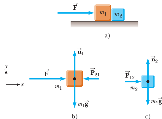
Figura 5.12 (Ejemplo 5.7). a) Se aplica una fuerza se a un bloque de masa m_1 , que empuja a un segundo bloque de masa m_2 . b) Diagrama de cuerpo libre para m_1 . c) Diagrama de cuerpo libre para m_2 .
