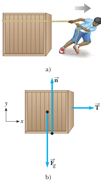
Figura 5.8 a) Una caja que se jala hacia la derecha sobre una superficie sin fricción. b) Diagrama de cuerpo libre que representa las fuerzas externas que actúan sobre la caja.
